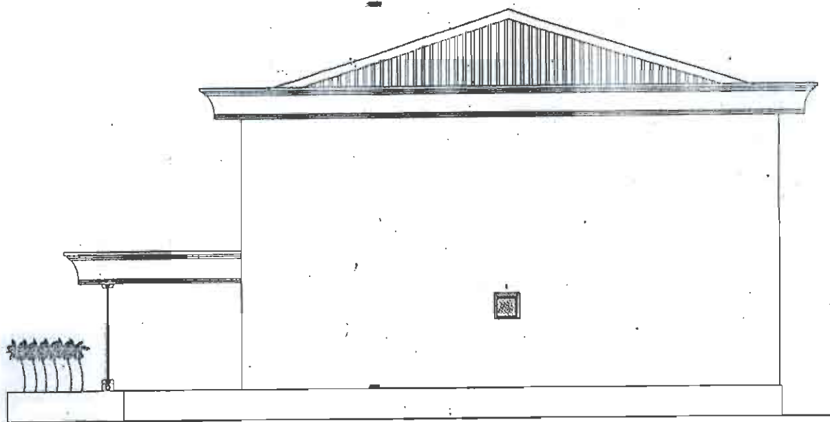
PIGNON GAUCHE
